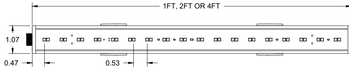
1 PLAN VIEW SCALE: 6"=1'-0"
