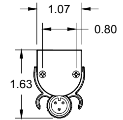
3 END CAP SCALE: 6"=1'-0"
