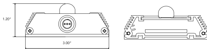
End Cap
