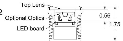
4 SECTION SCALE: 6"=1'-0"
