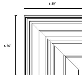
KEC Profile
