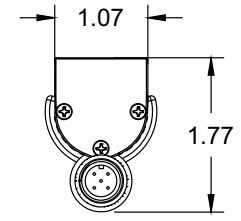
3 END CAP SCALE: 6"=1'-0"
