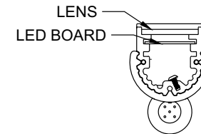
4 SECTION SCALE: 6"=1'-0"
