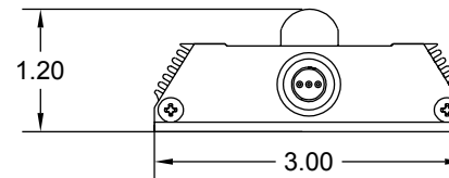
3 END CAP SCALE: 6"=1'-0"
