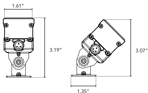
Swivel
