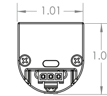
3 END CAP
