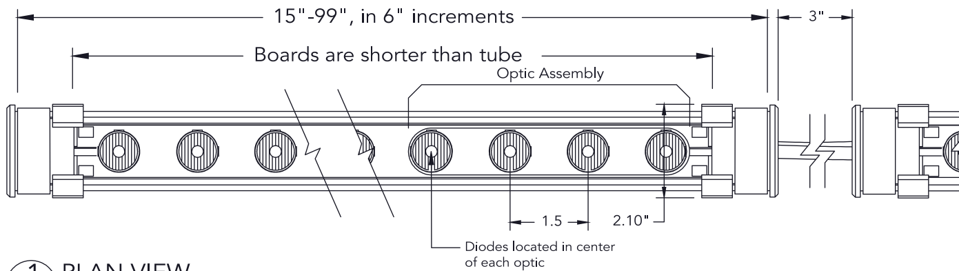
1 PLAN VIEW SCALE: 6" = 1'-0"
