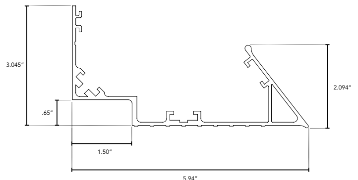
KEC Profile
